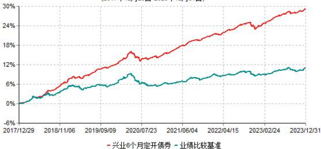
兴业6个月定期开放债券型发起式证券投资基金累计净值增长率与业绩比较基准收益率历史走势对比图 (2017年12月29日-2023年12月31日)
